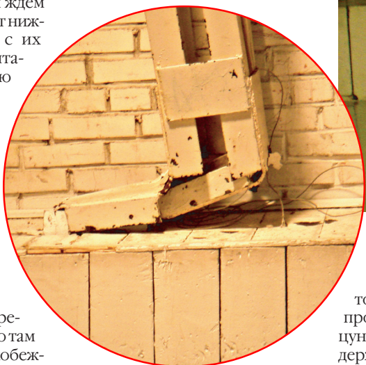
«Подломленная» опора фермы
