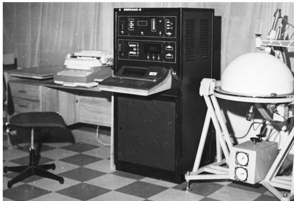
Стенд «Импульс-5»
